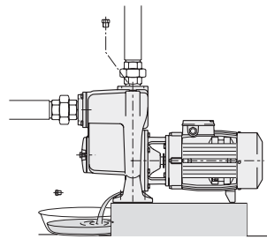
Fig. 3 Scarico Draining Entleerung Vidange Vaciado Vacío Avtappning Aftappen Αποστράγγιση Слив 排泵
